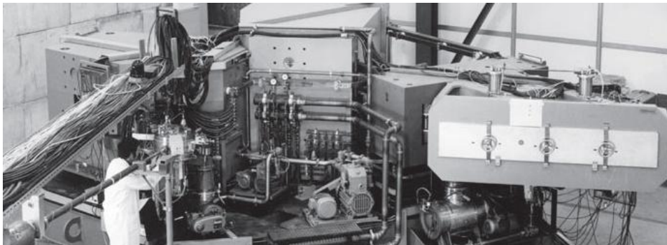
Großer Massenspektrograph mit 3 Dipol- und einem Quadrupolmagneten.
