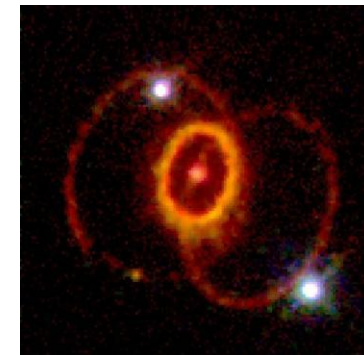
Überrest der Supernova 1987A, die 1987 durch sichtbares Licht und erstmals auch durch Neutrinos nachgewiesen wurde.
